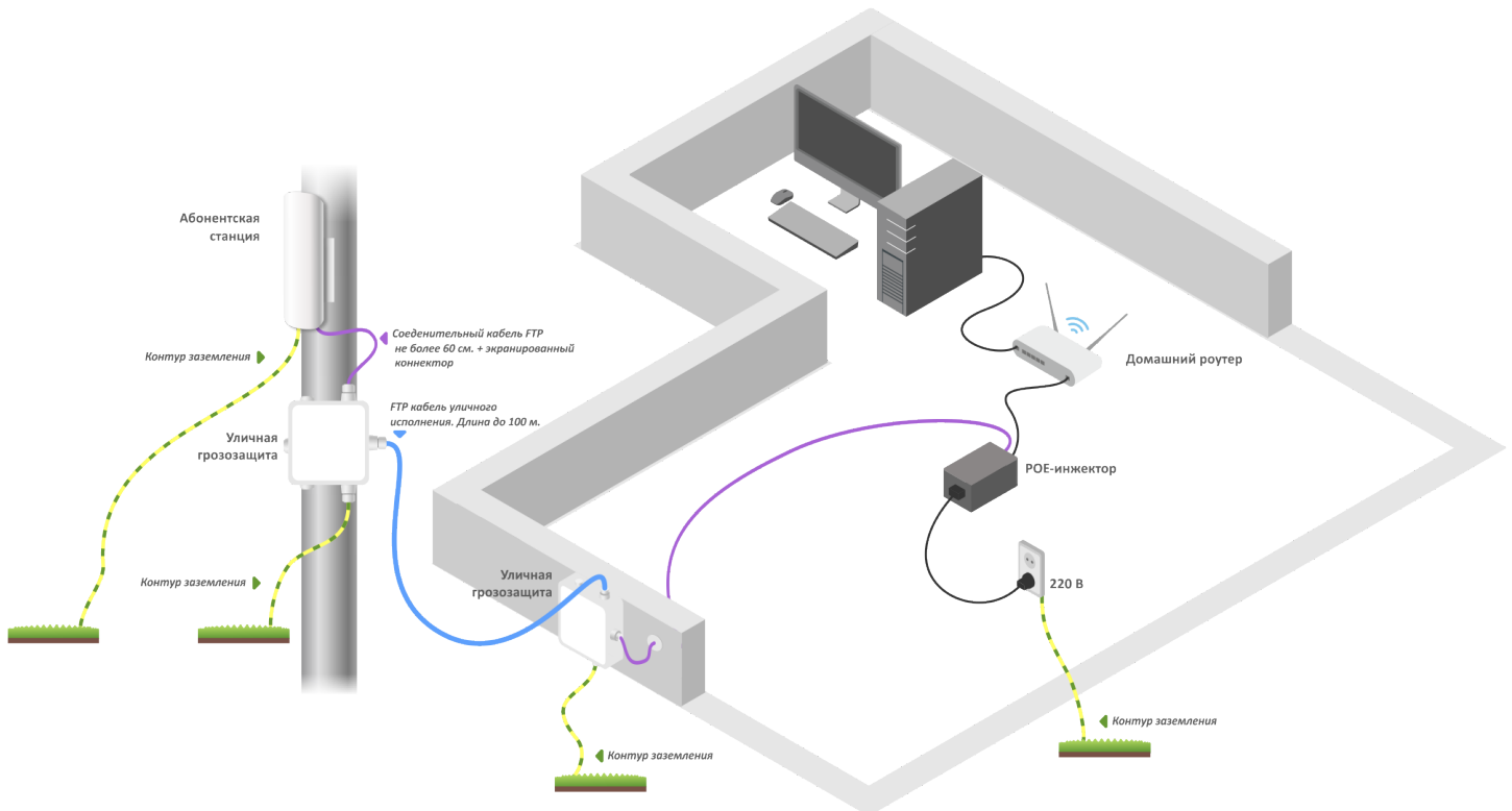
Схема подключения абонентской станции для обеспечения грозозащиты
