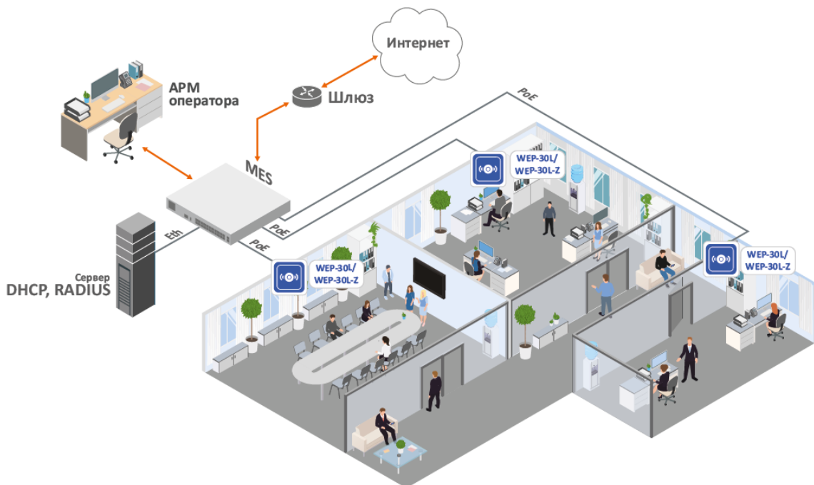
Рисунок 1 — Функциональная схема использования WEP-30L/WEP-30L-Z
