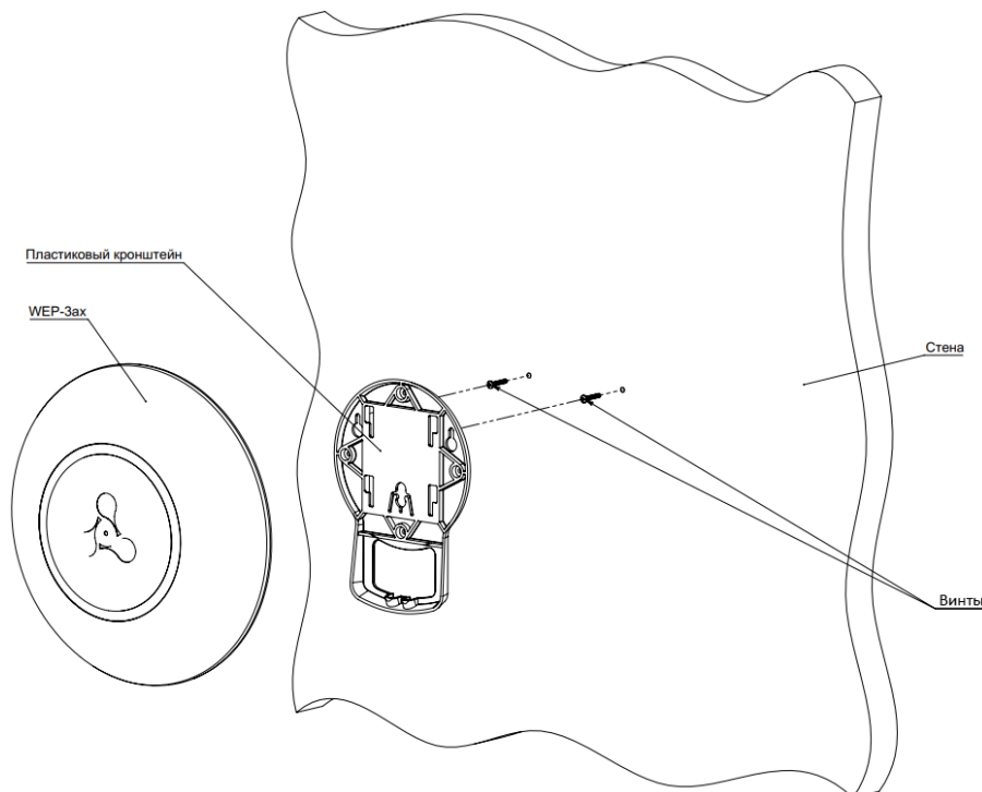
Рисунок 8 — Крепление кронштейна на стене
